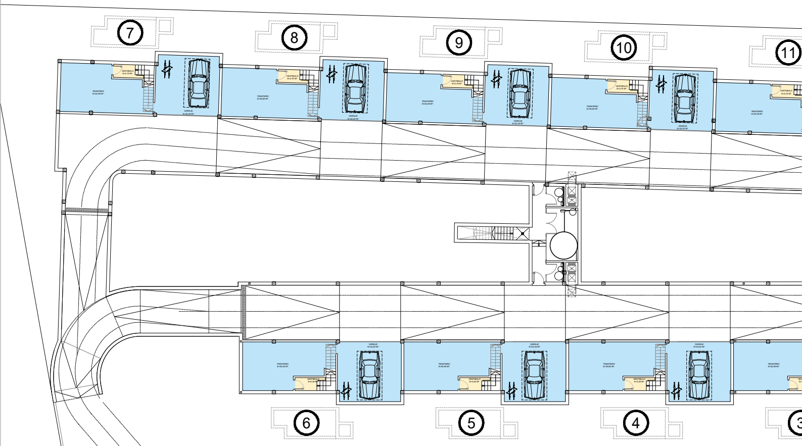
PLANTA SOTANO
