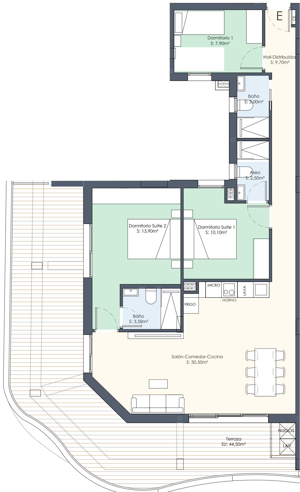
Planta Vivienda
