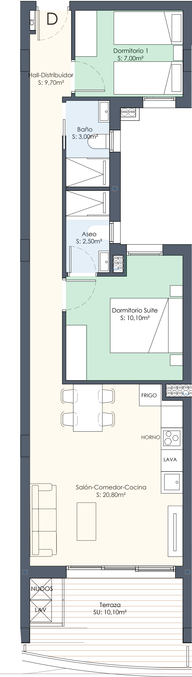
Planta Vivienda
