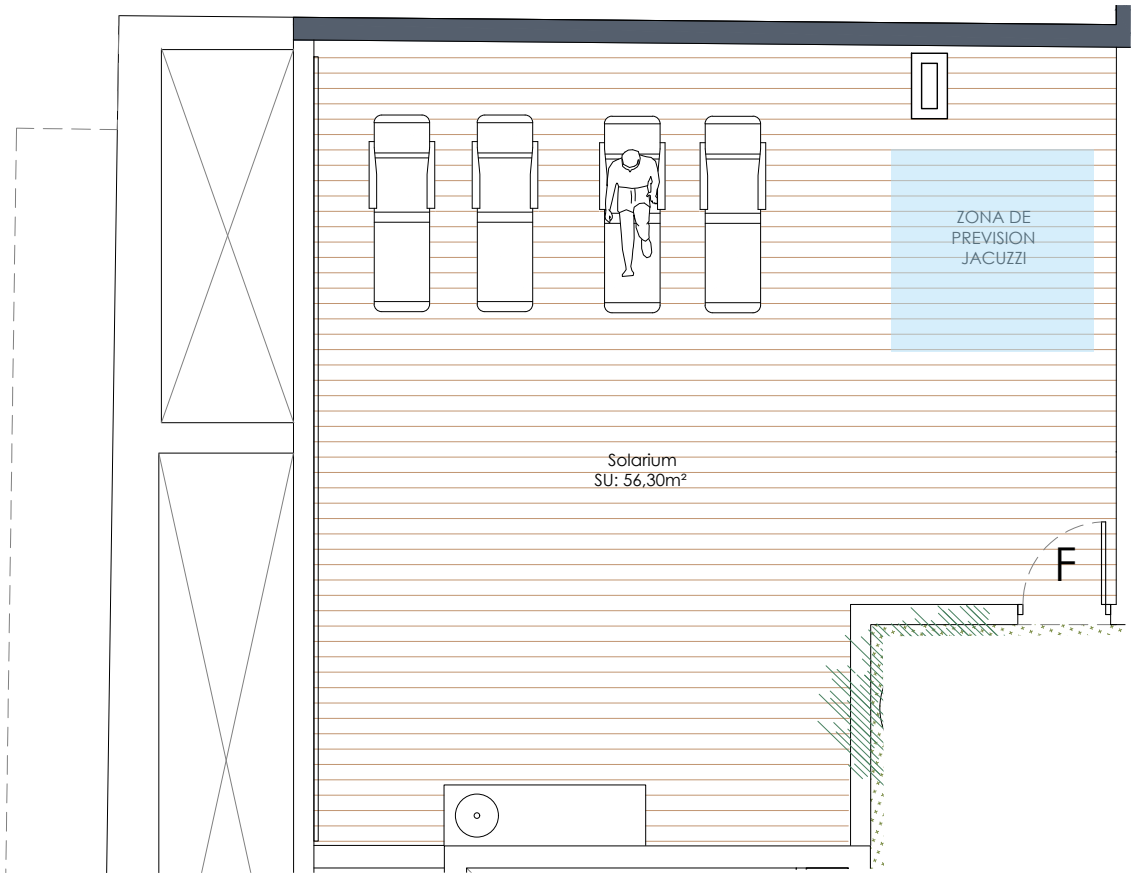
Planta Solarium
