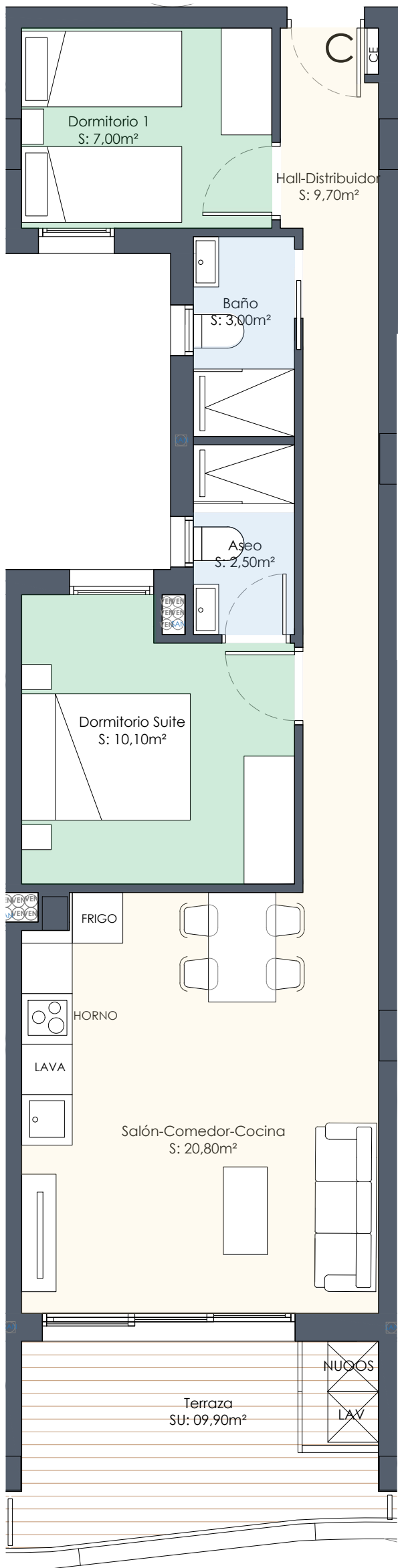
Planta Vivienda
