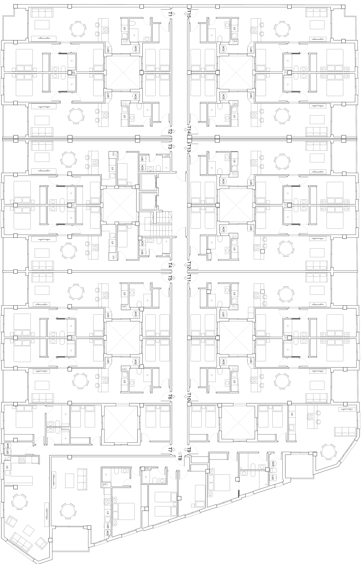
Planta Segunda
