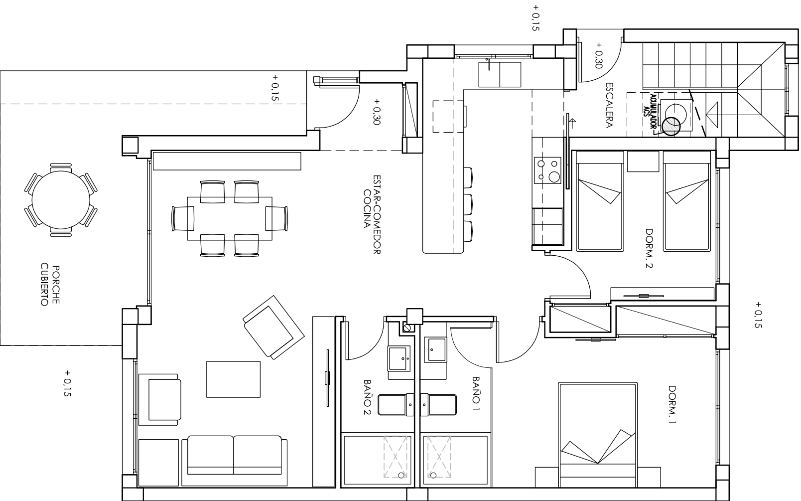
PLANTA BAJA
