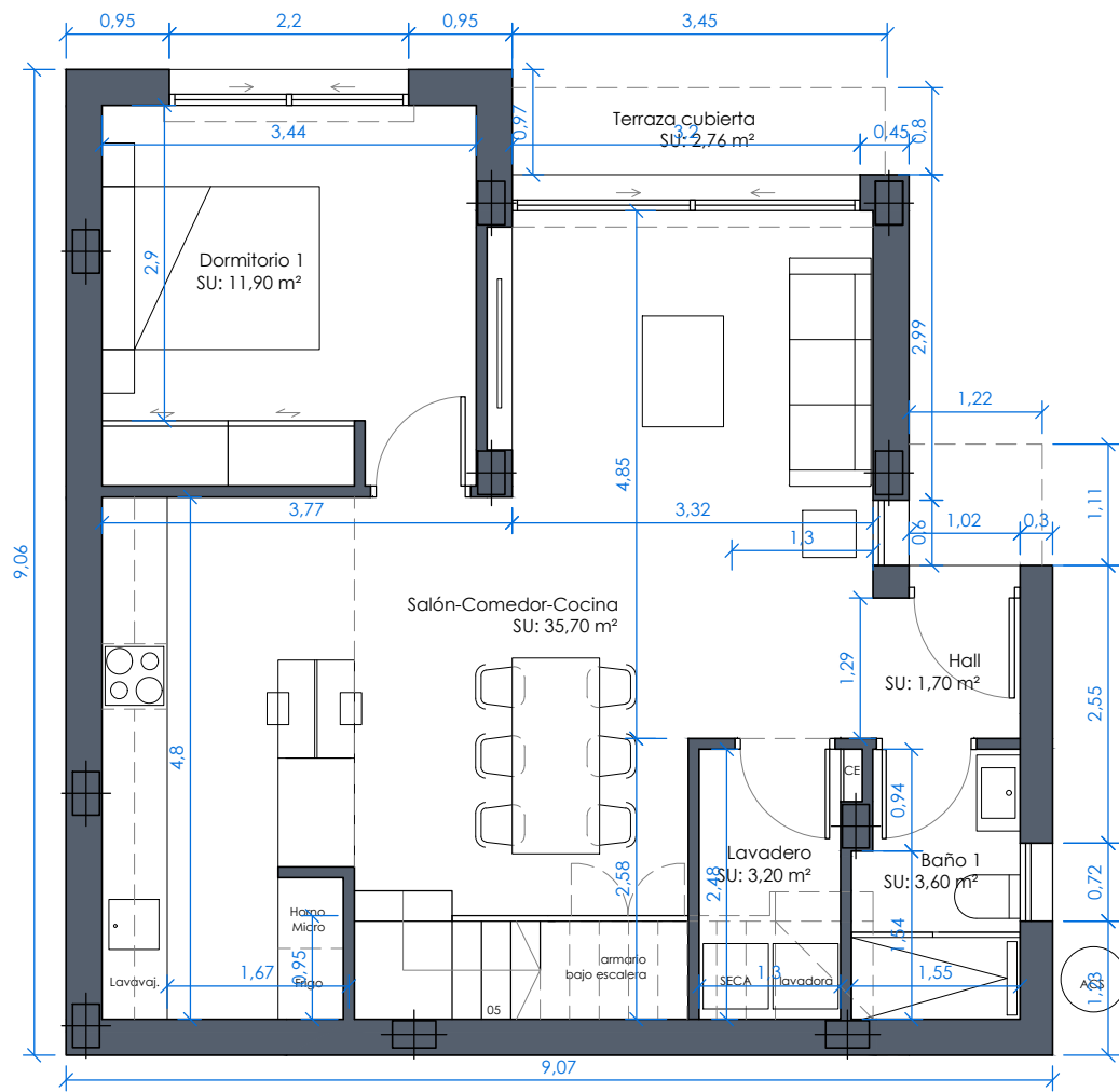
PLANTA BAJA
