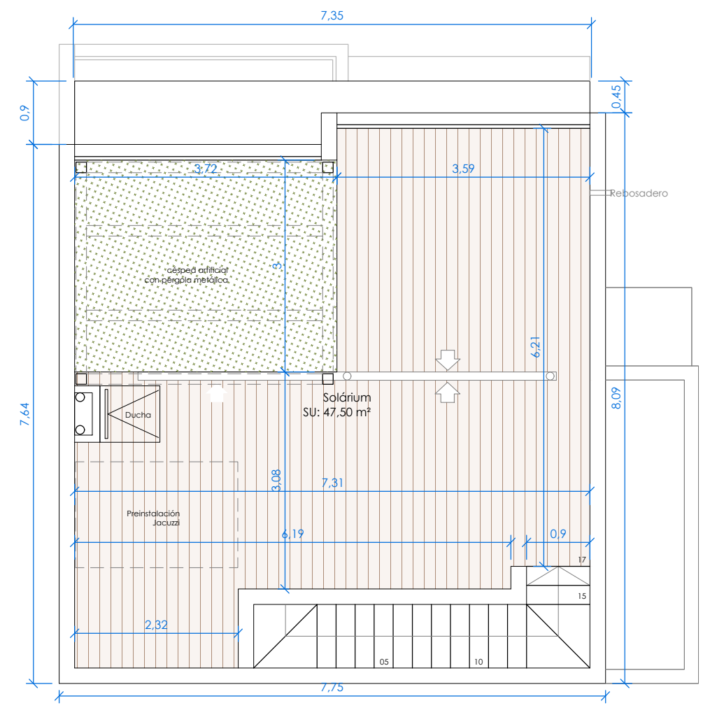
PLANTA CUBIERTA
