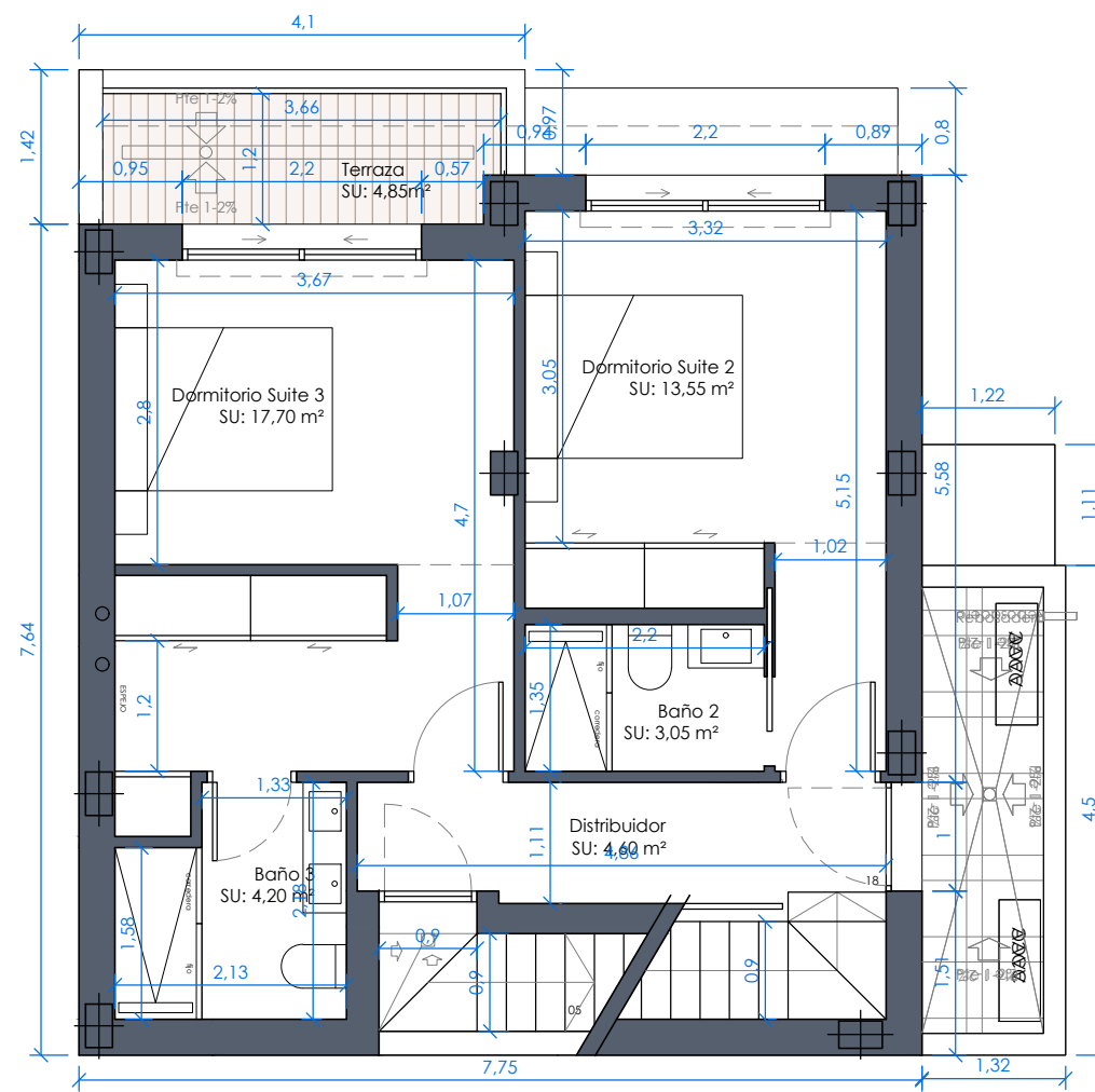
PLANTA PRIMERA
