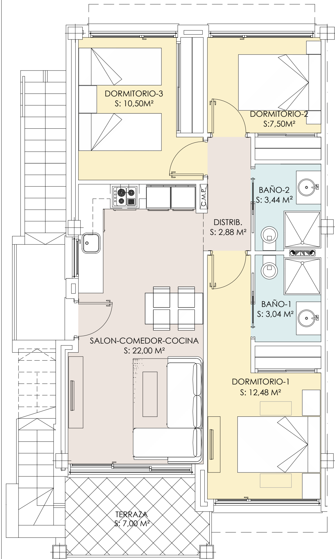
PLANTA PRIMERA
