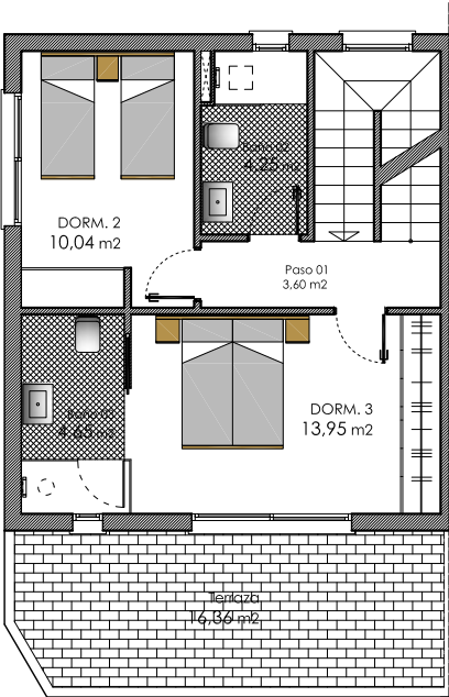
PLANTA PRIMERA
