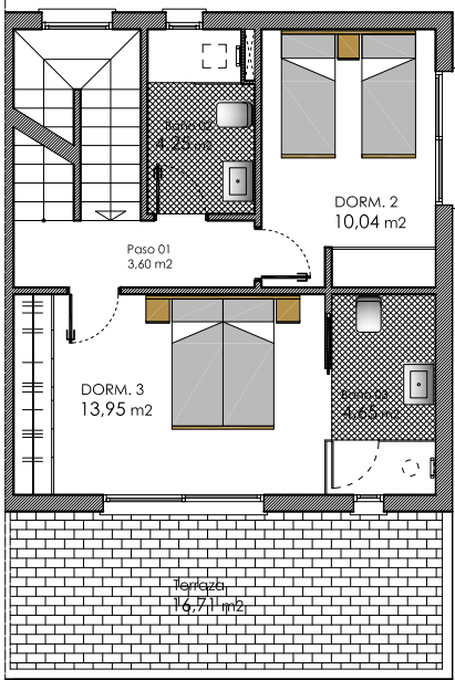
PLANTA PRIMERA
