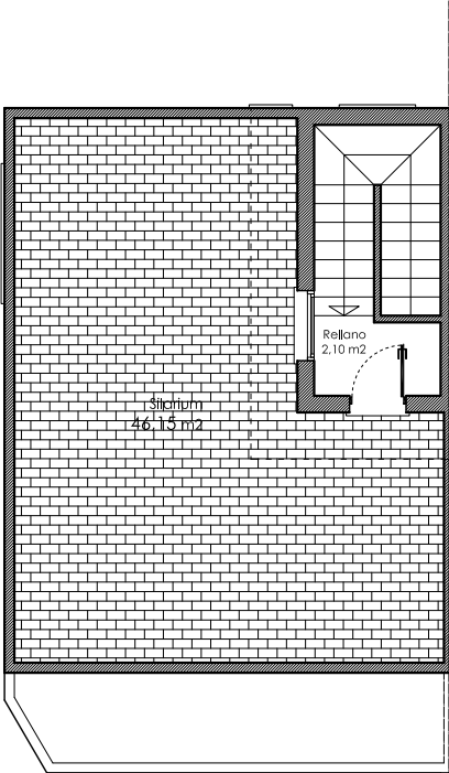
PLANTA SOLARIUM
