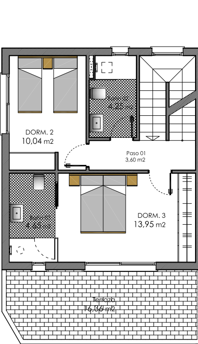
PLANTA PRIMERA
