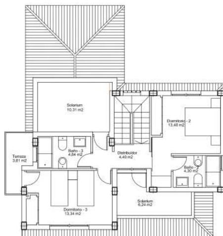
PLANTA PRIMERA ESCALA: 1 / 100
