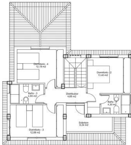
PLANTA PRIMERA ESCALA: 1 / 100
