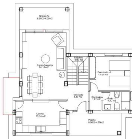
PLANTA BAJA ESCALA: 1 / 100
