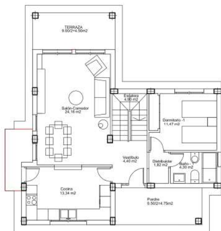
PLANTA BAJA ESCALA: 1 / 100
