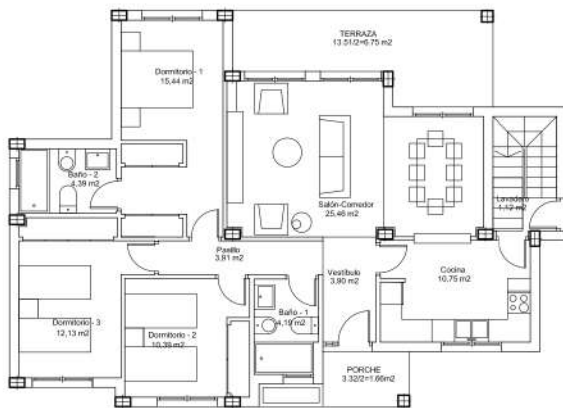
PLANTA BAJA ESCALA: 1 / 100
