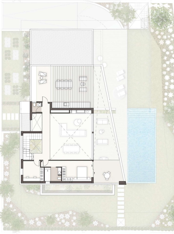
PLANTA PRIMERA
