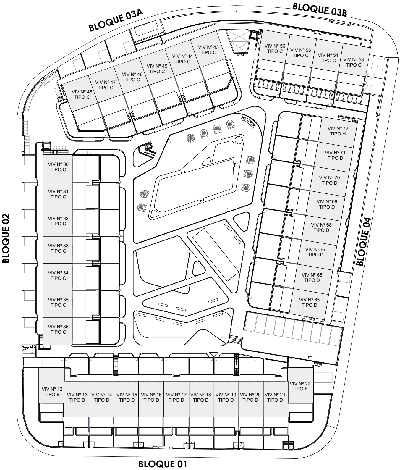
PLANTA PRIMERA Y SEGUNDA
