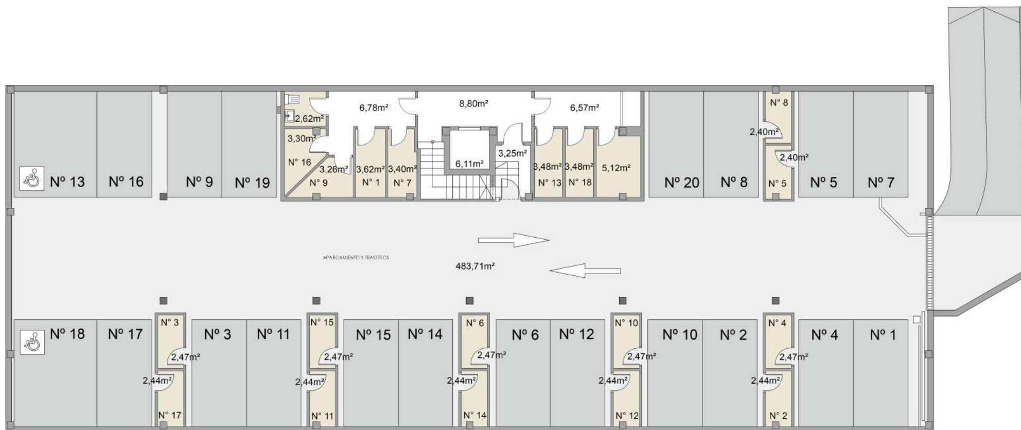
BLOQUE 1 Planta sótano
