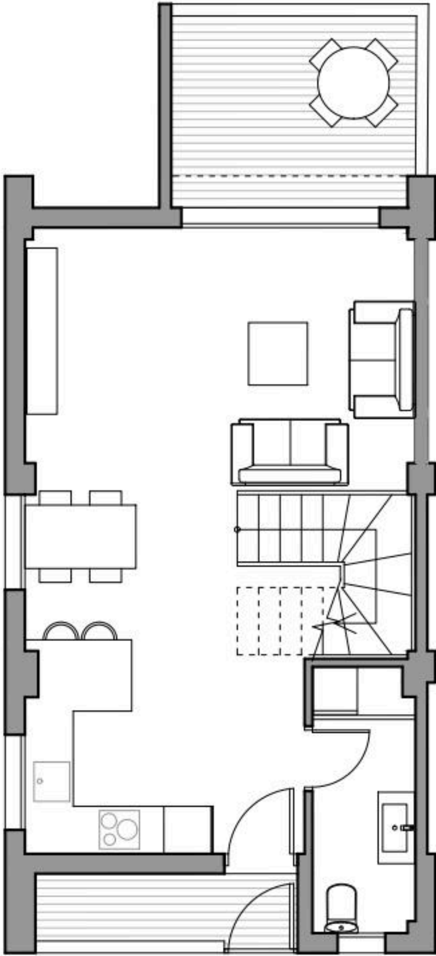
PLANTA BAJA
