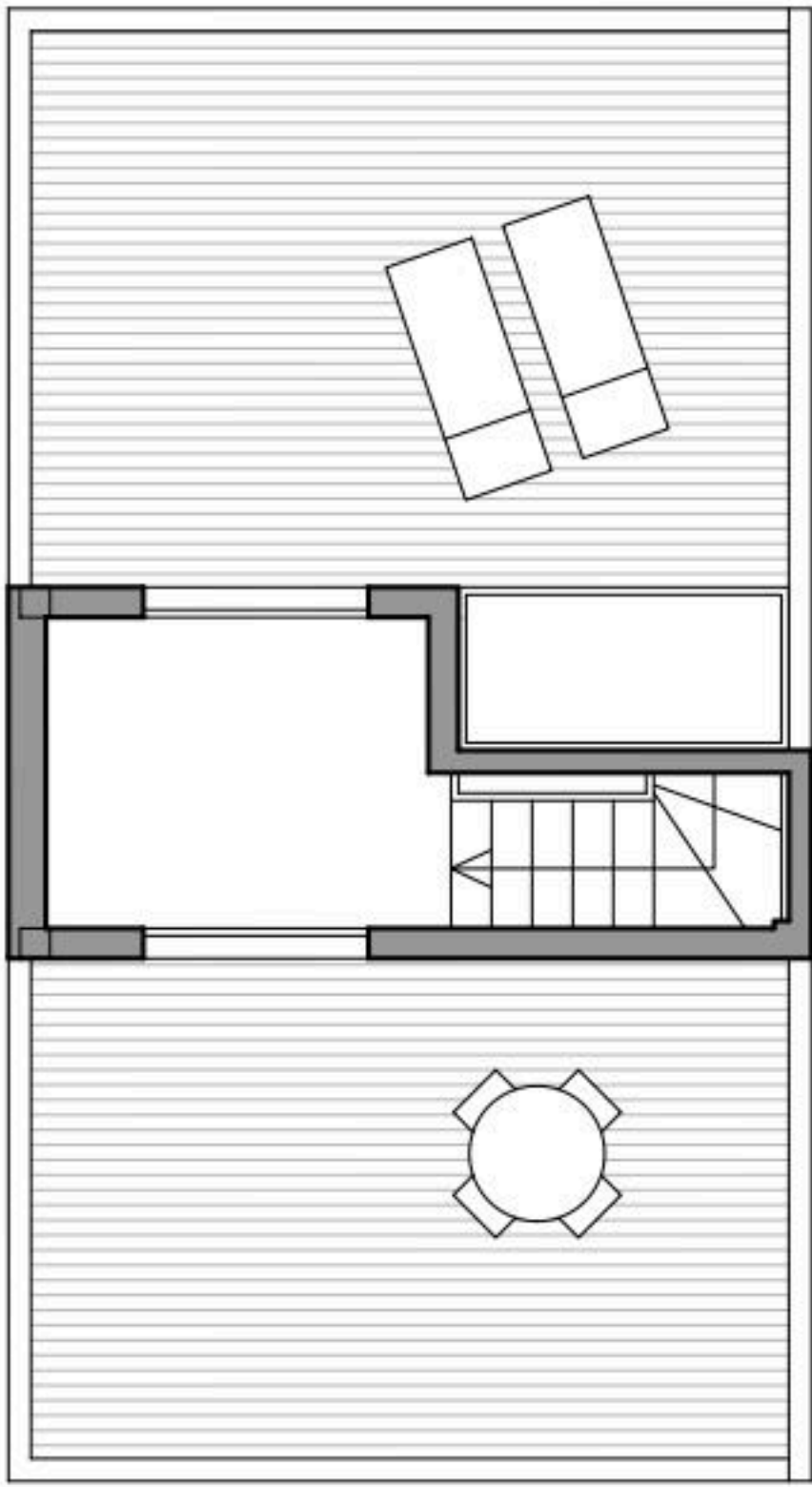
PLANTA CUBIERTA
