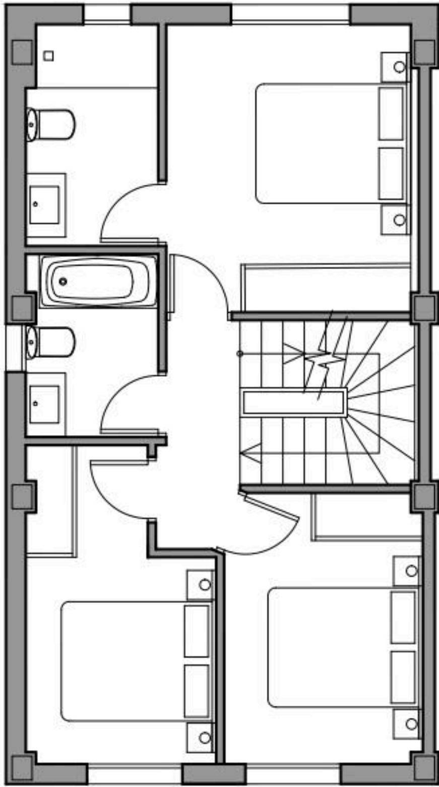
PLANTA PRIMERA
