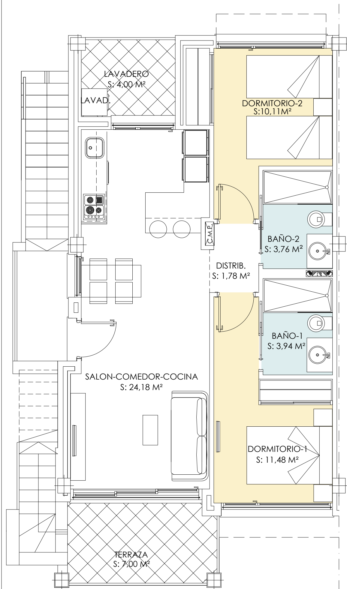
PLANTA PRIMERA
