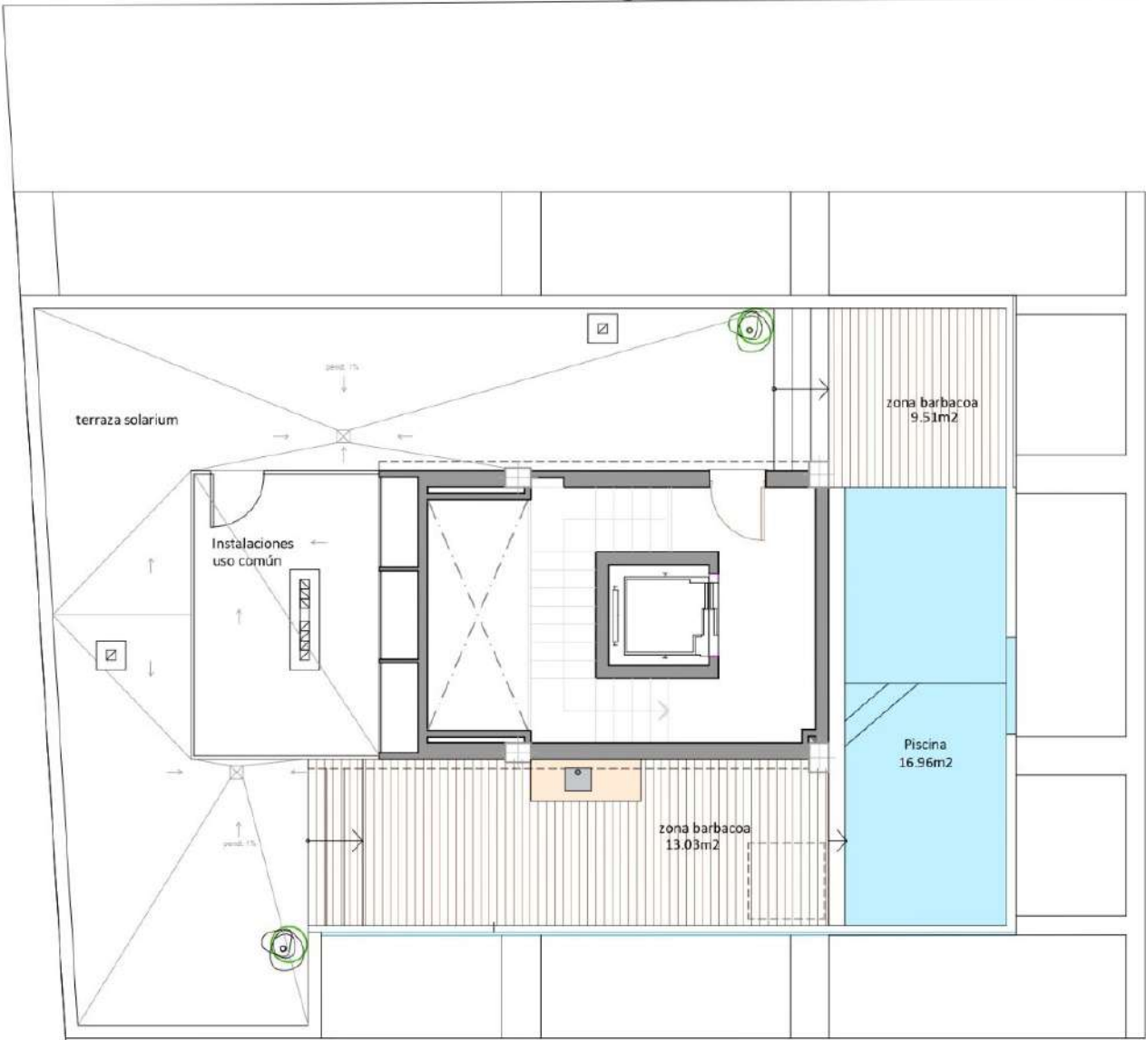
PLANTA CUBIERTA (SOLARIUM Y PISCINA)
