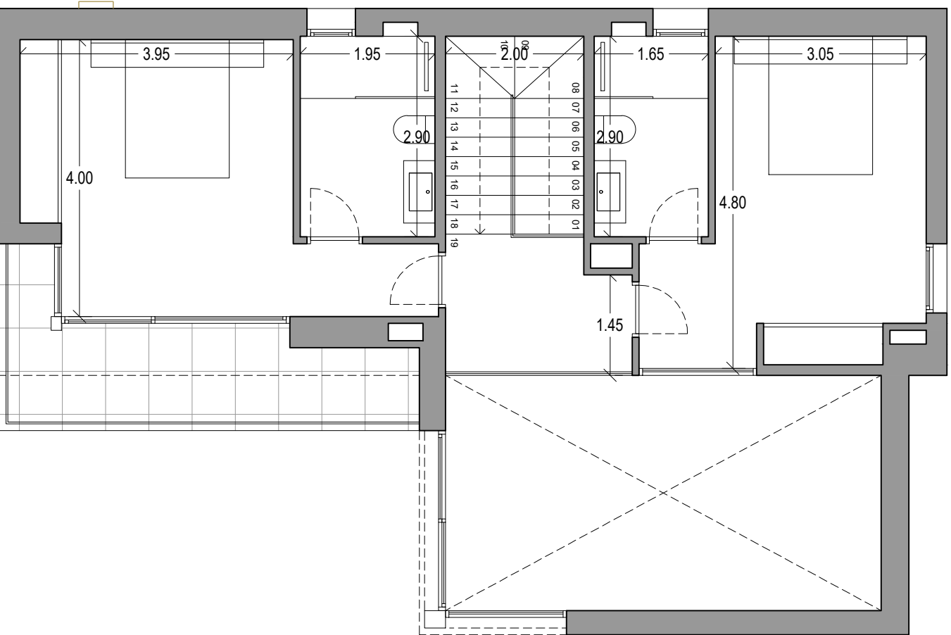
PLANTA ALTA - COTAS
