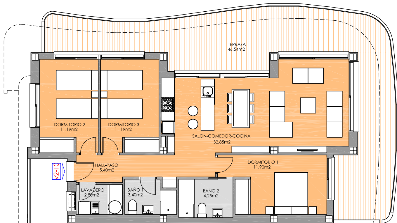
bloque 1 planta segunda
