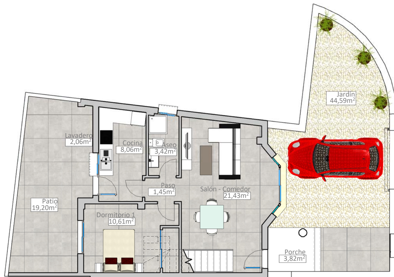
PLANTA BAJA
