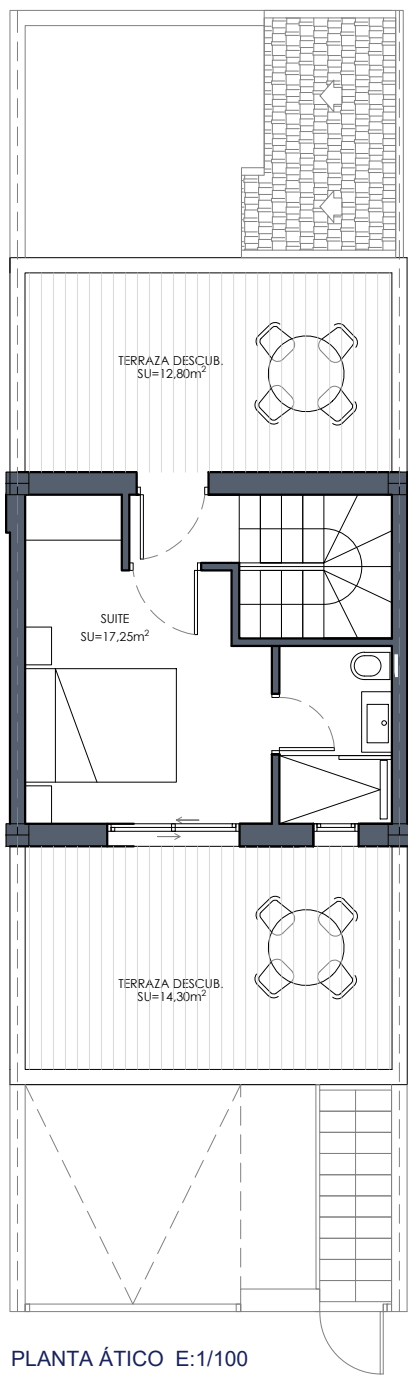
PLANTA ÁTICO E:1/100
