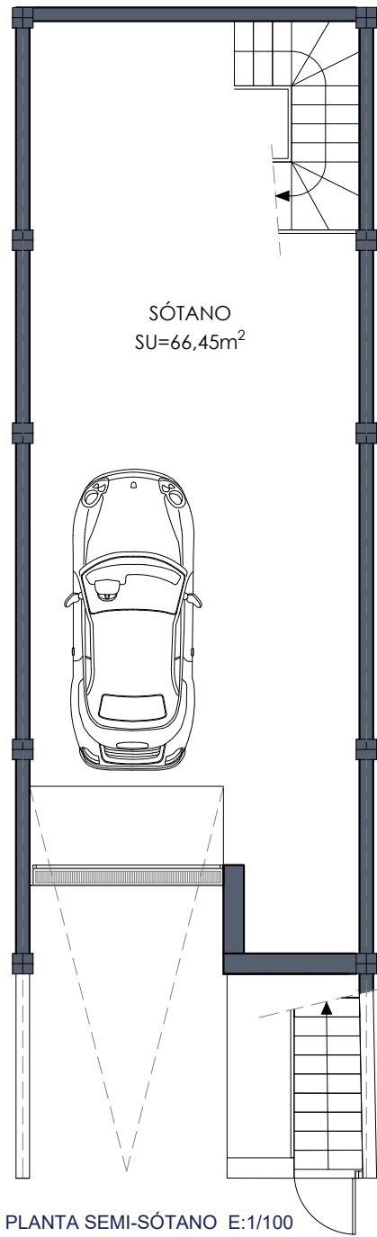
PLANTA SEMI-SÓTANO E:1/100
