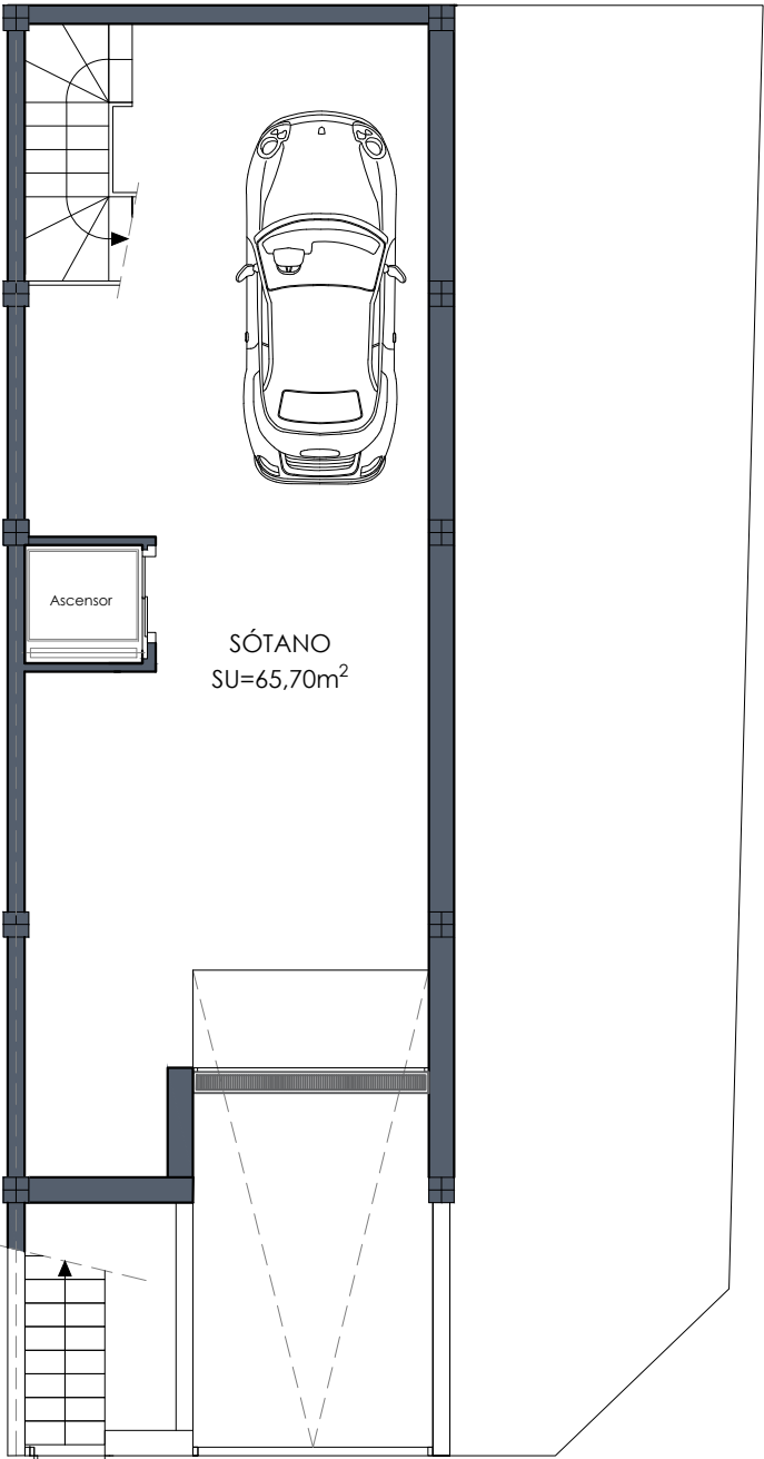
PLANTA SEMI-SÓTANO E:1/100
