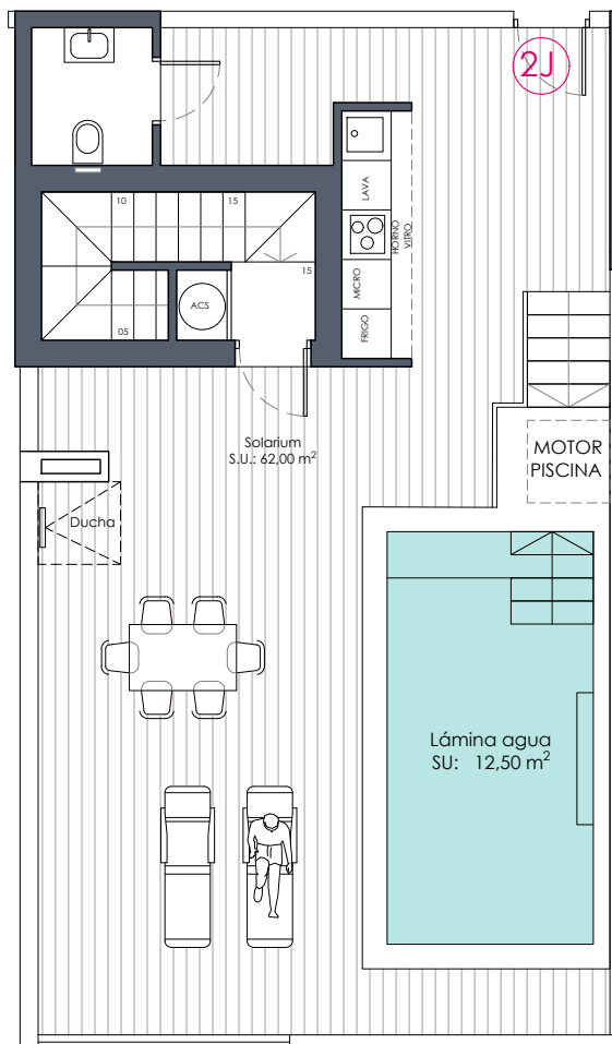
Planta Solarium
