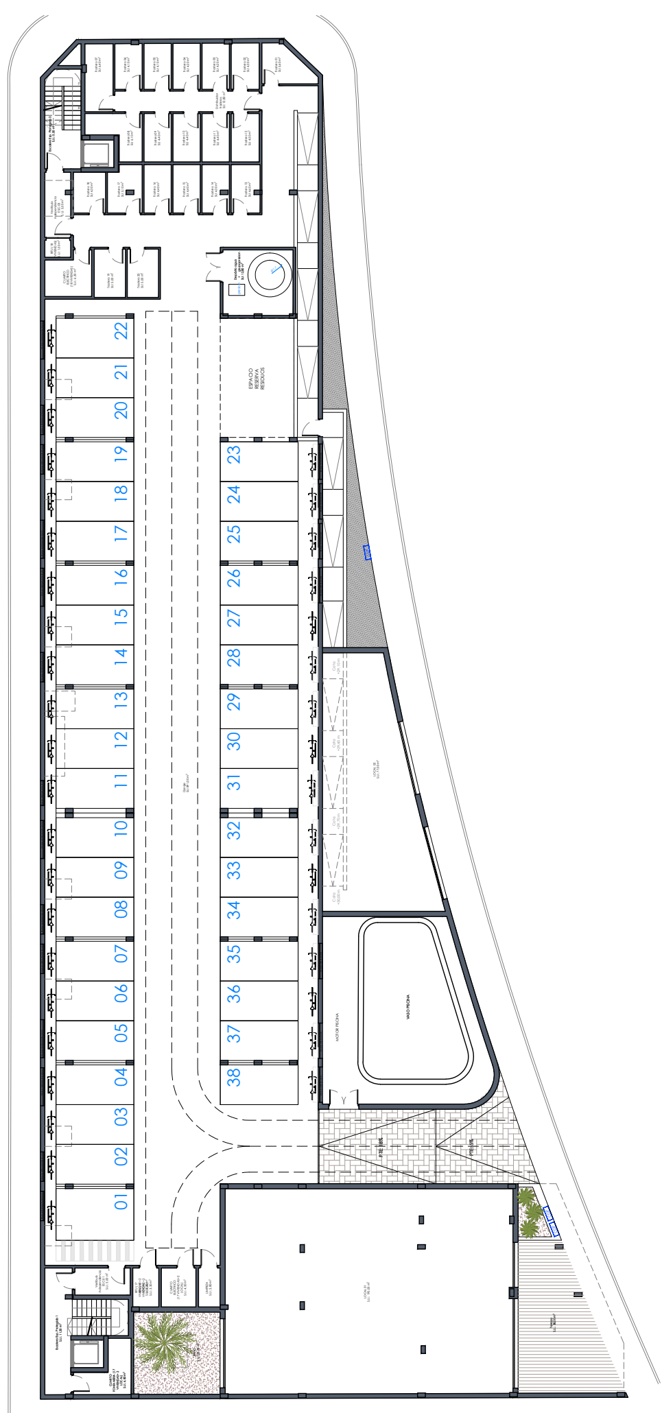
Planta Sótano -1
