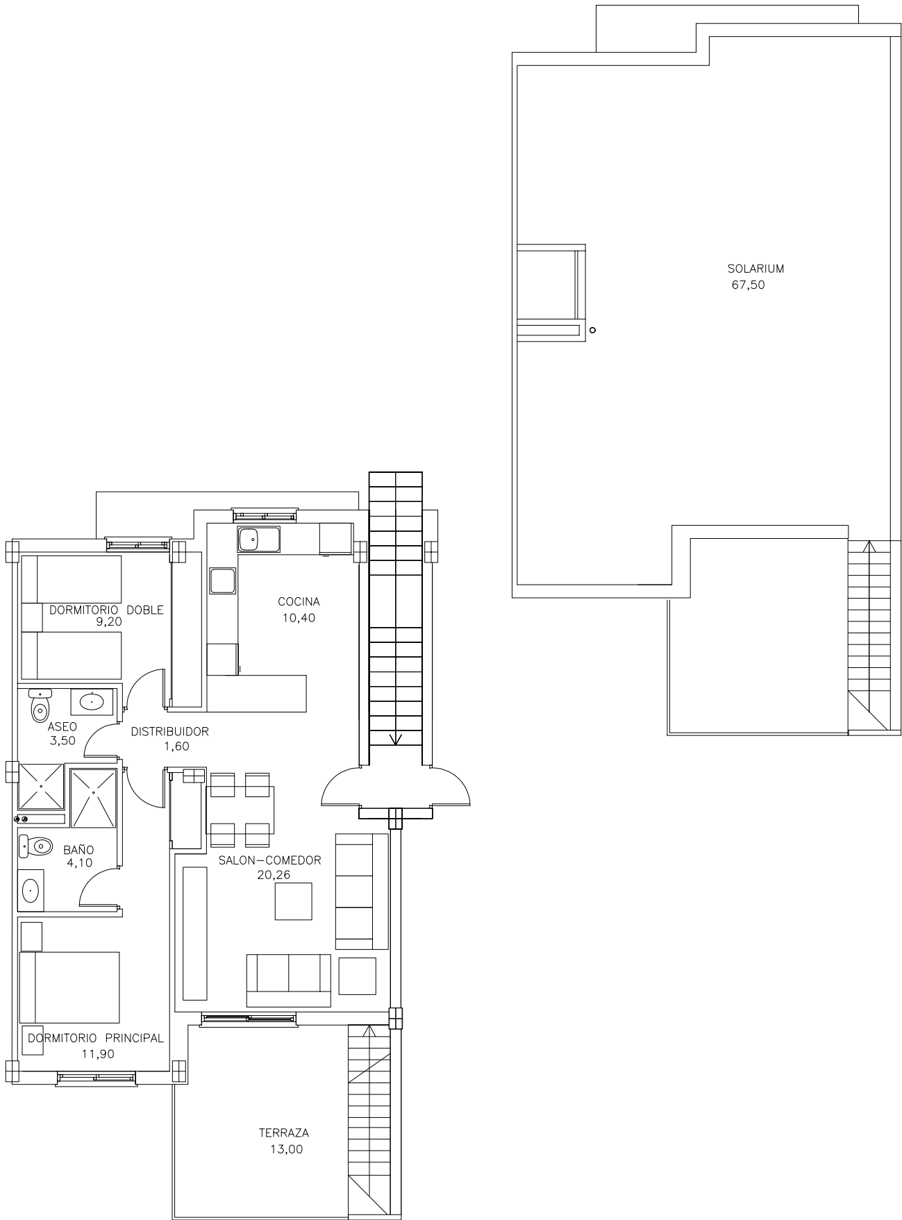
VIVIENDA 4
