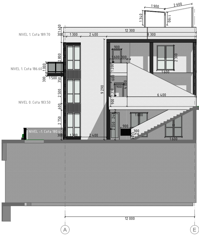
ALZADO DERECHO
