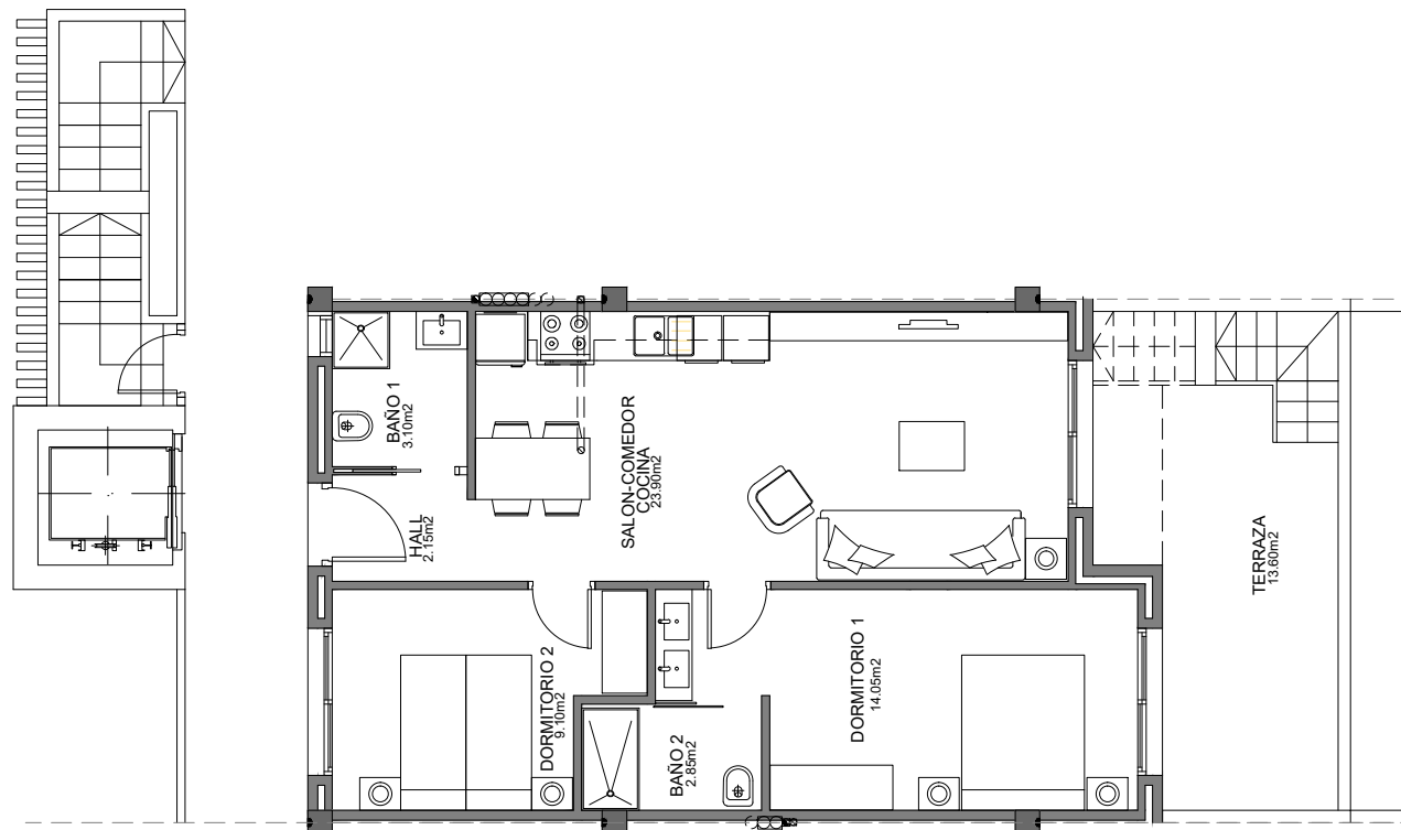
Planta Segunda
