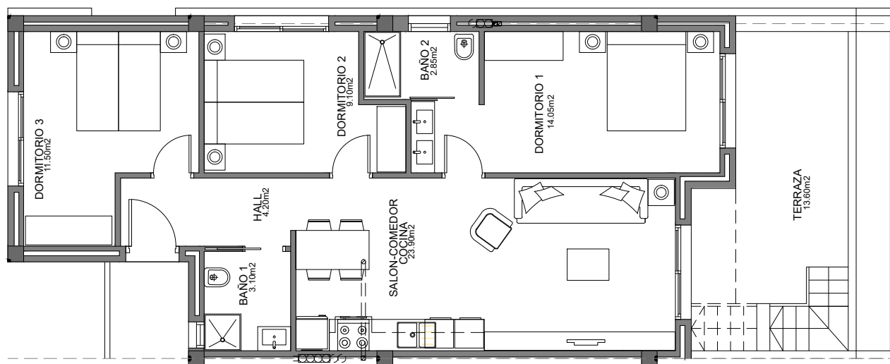
Planta Segunda
