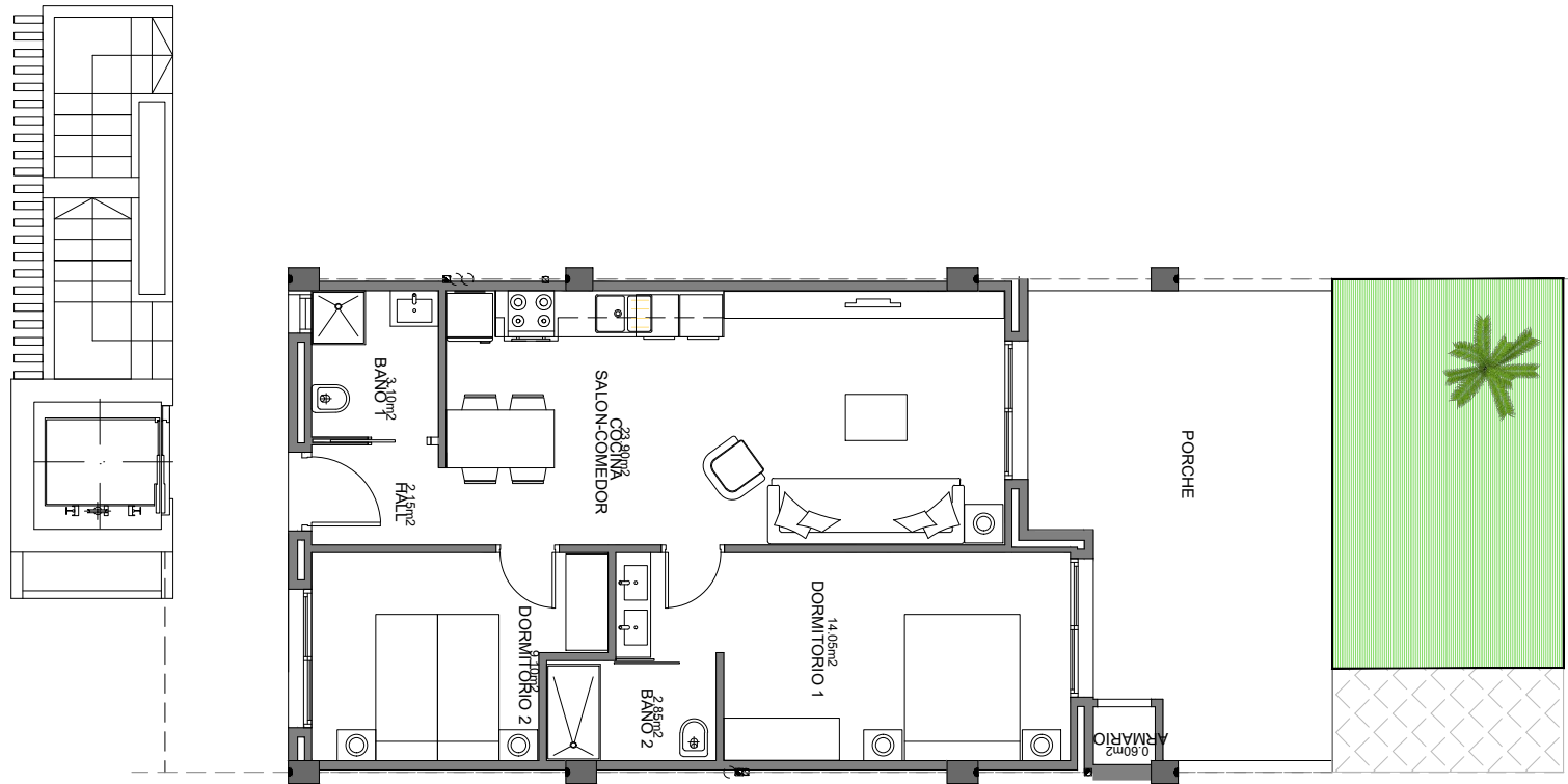
Planta Baja
