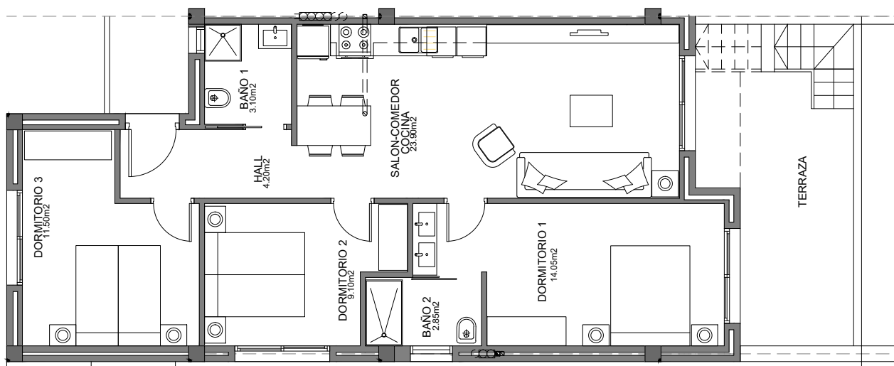
Planta Segunda
