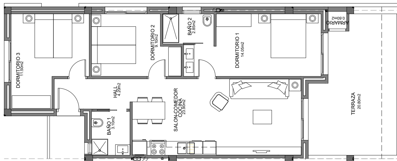
Planta Primera
