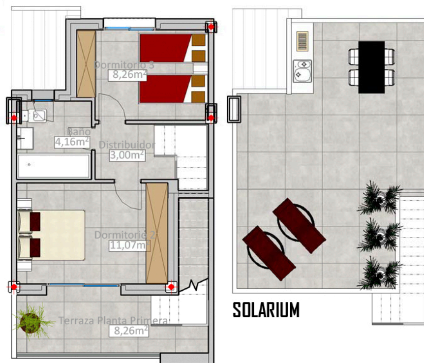
PLANTA PRIMERA
