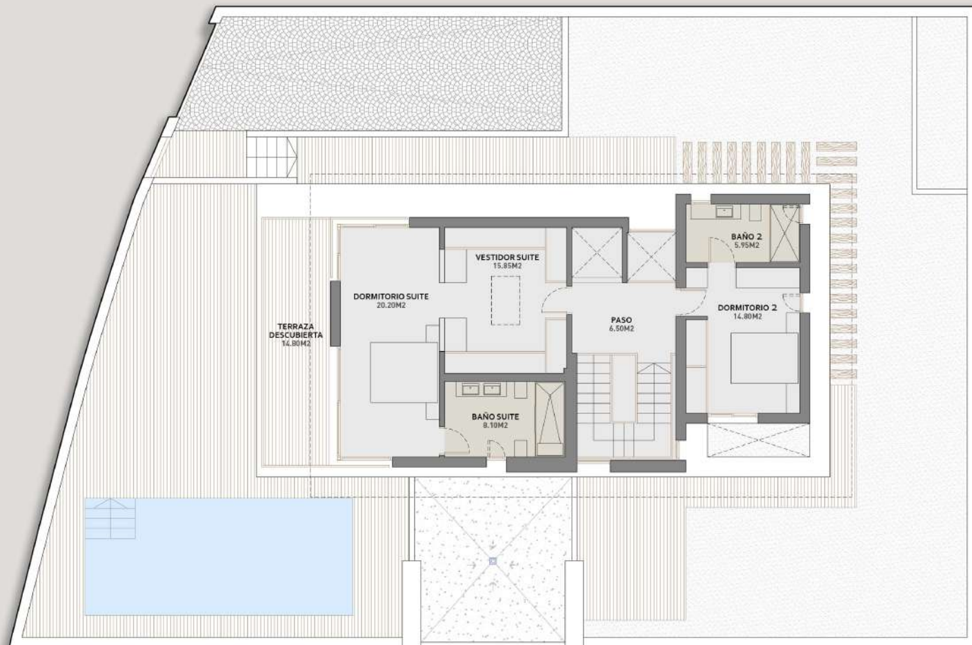
PLANTA ALTA
