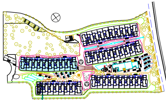
bloque 1 ordenacion general
