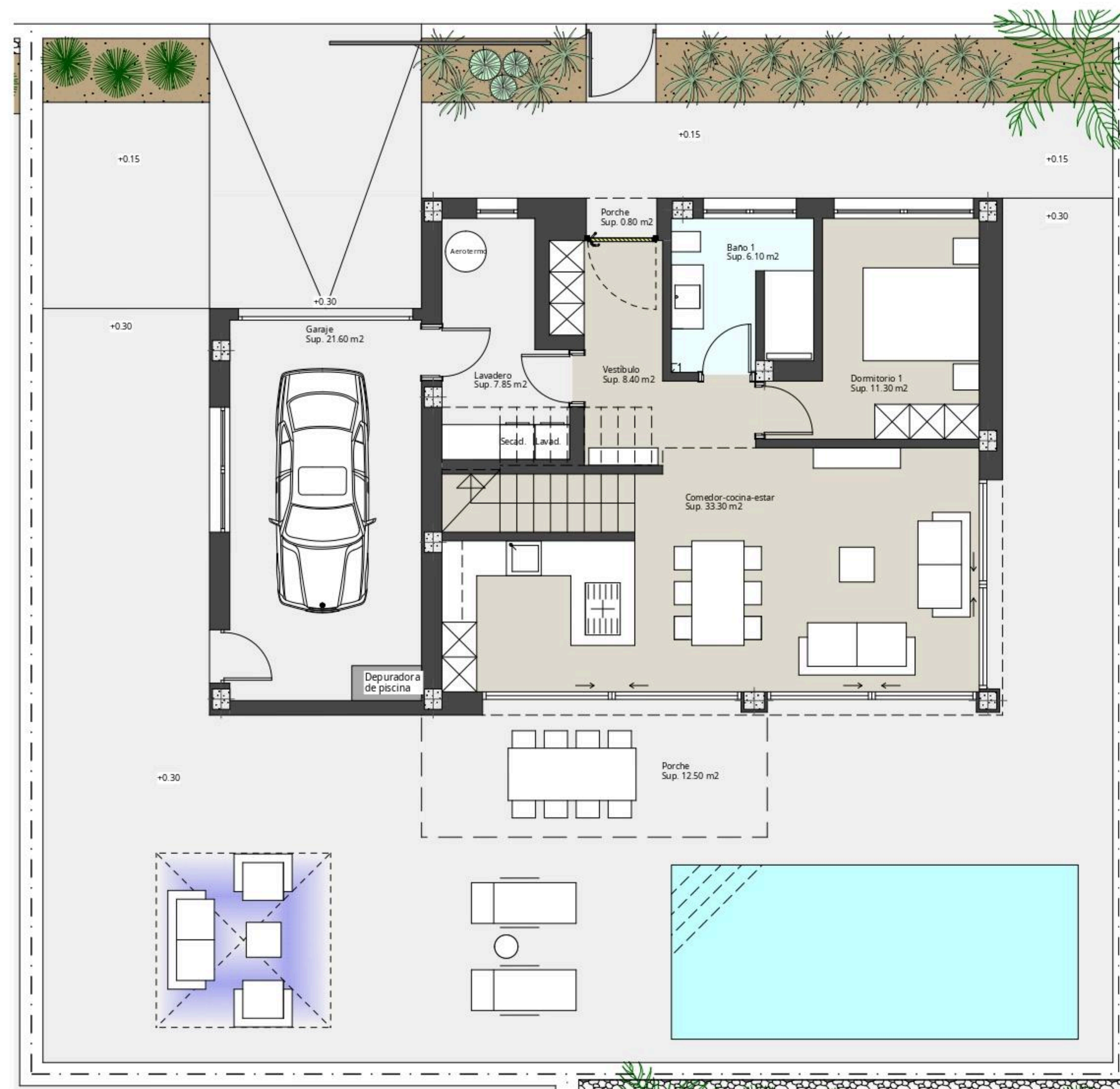
Planta baja
